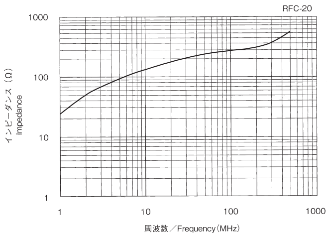
インピーダンス周波数特性*
