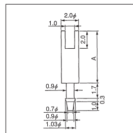
KSタイプ (取付穴1.0φ用)
