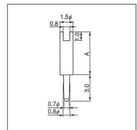
KBタイプ (取付穴0.8φ用)
